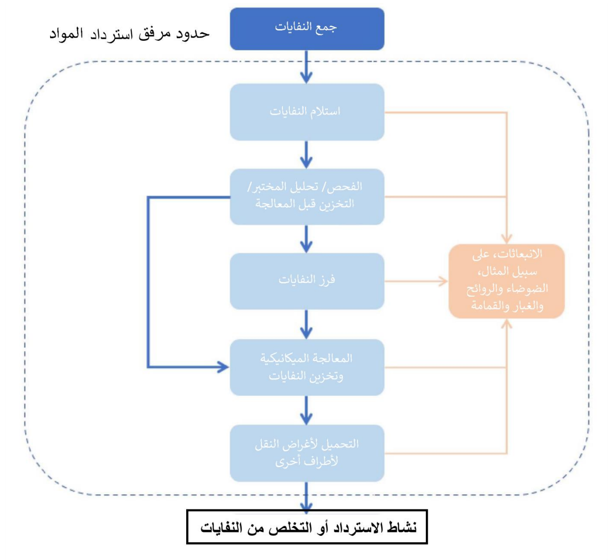
الشكل 1-4 التسلسل العام لمعالجة النفايات في مرفق استرداد المواد.
