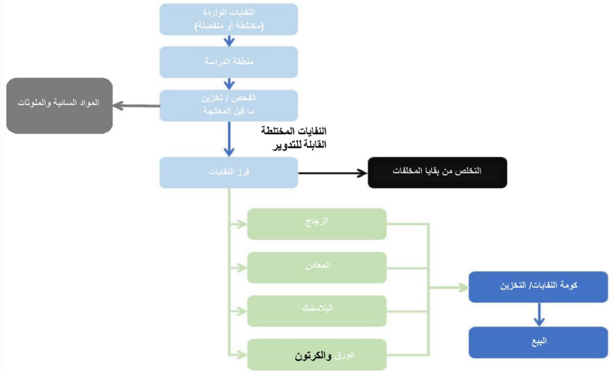
الشكل 4-3: تسلسل عمليات معالجة نفايات بمرفق استرداد المواد النظيفة.
