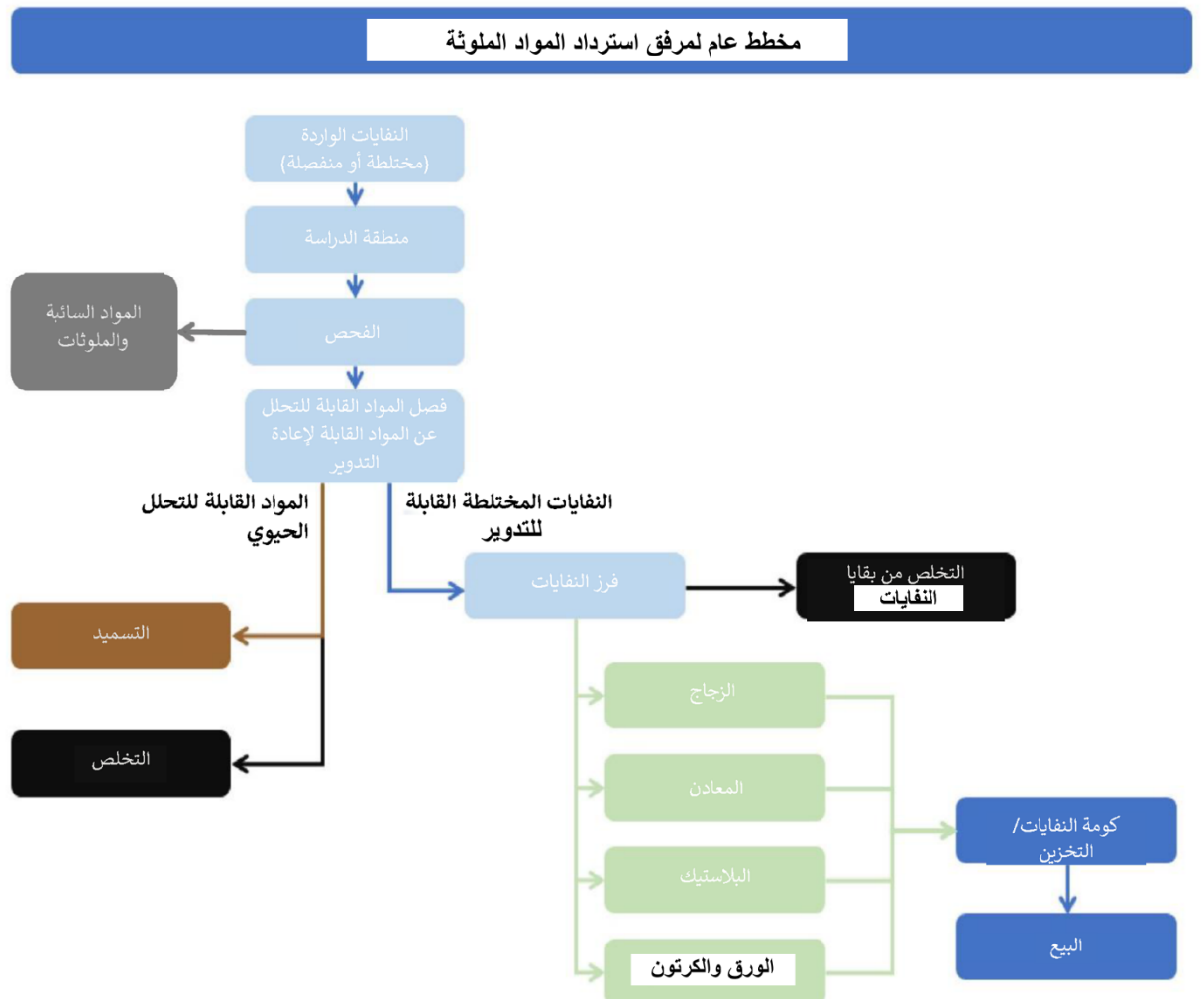
الشكل 2-4: تسلسل عمليات معالجة نفايات مرافق استرداد المواد الملوثة.
